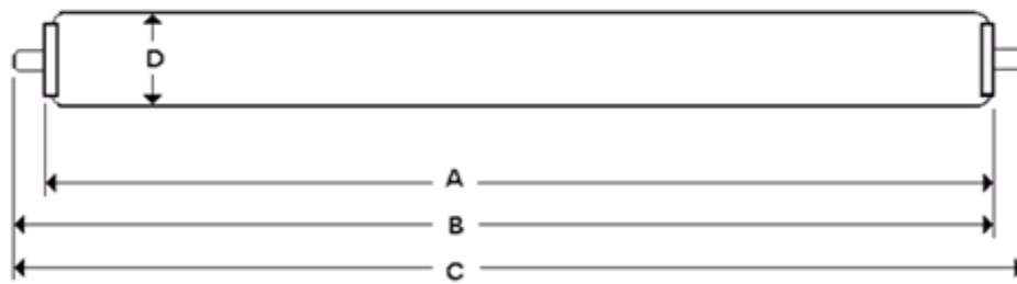
Figura B2: Dimensiones de la lámpara con casquillo Fa8
