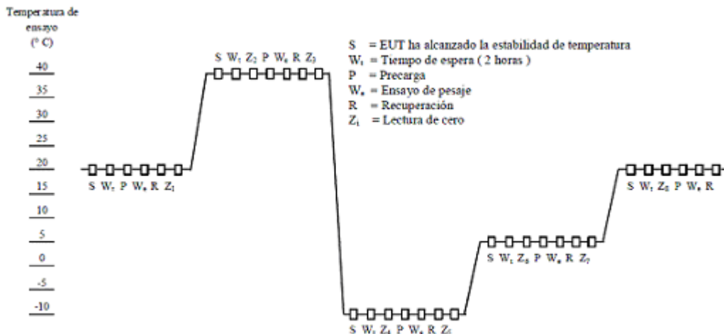
Figura A.3-Secuencia de prueba propuesta para la prueba A.5.3.1 combinado con A.5.3.2 (prueba de temperatura cuando los límites de temperatura son + 40 °C / - 10 °C
