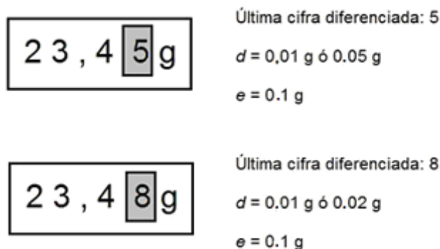
Figura 5-Ejemplo de dispositivos indicadores con una división de escala diferenciada
