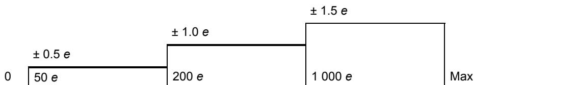
Figura 6-Errores máximos permitidos (emp) para la verificación inicial
